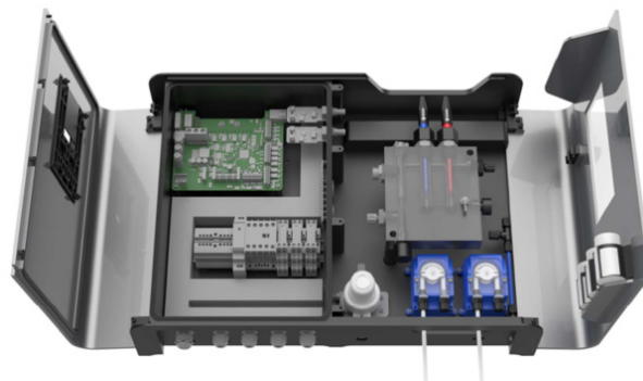
Offenes Gehäuse
