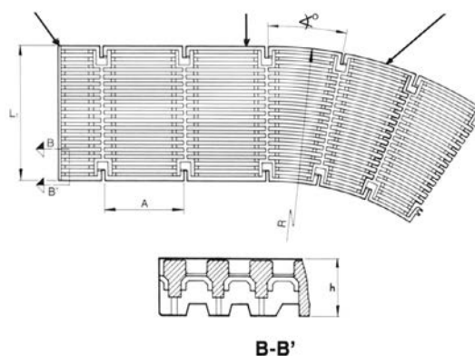
ENDSTÜCK
